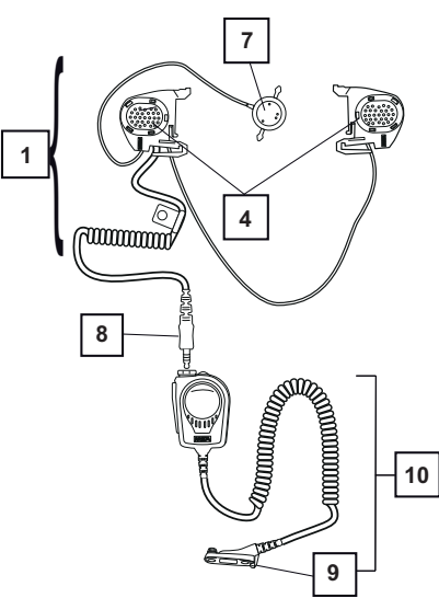
Figura 2 Cuffia a conduzione ossea
