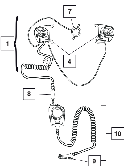
Abbildung 2 Körperschallleitende Sprechgarnitur
