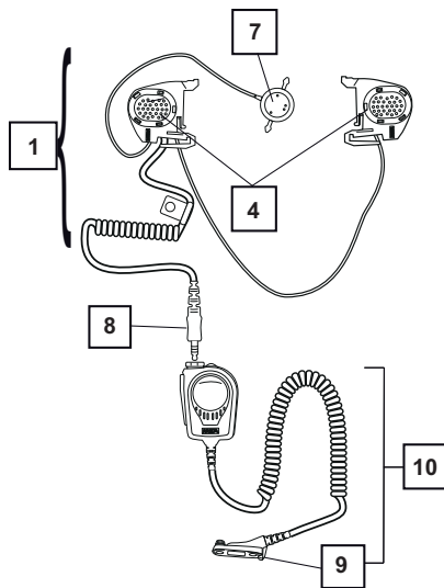
Ábra 2 Csontrezgéses fejhallgató
