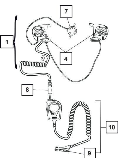
Figur 2 Beinledende hodesett
