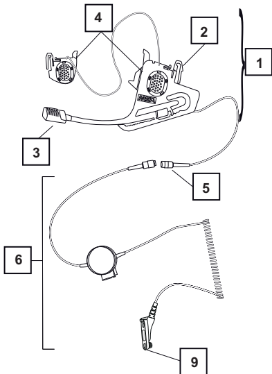
Kuva 1 Taipuisa kuulokemikrofoni
